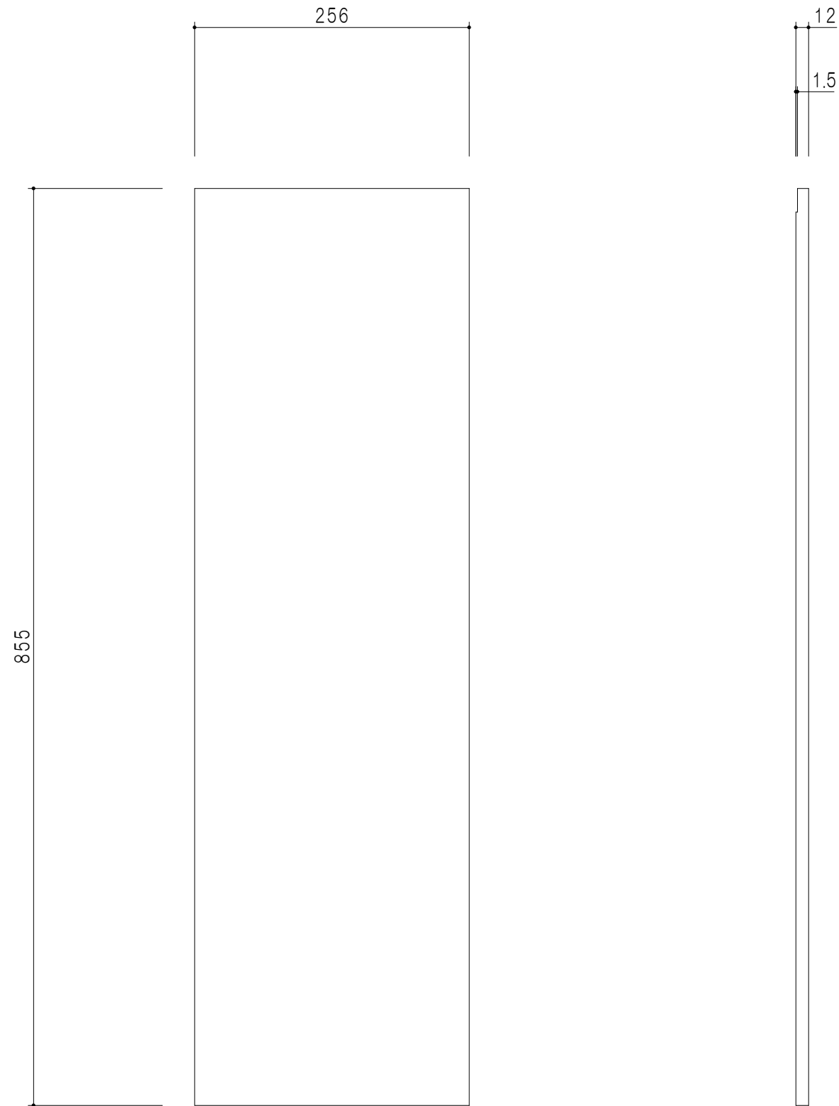
側面図
