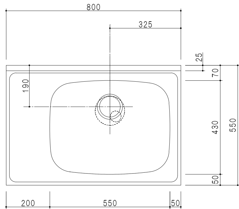
平面図
