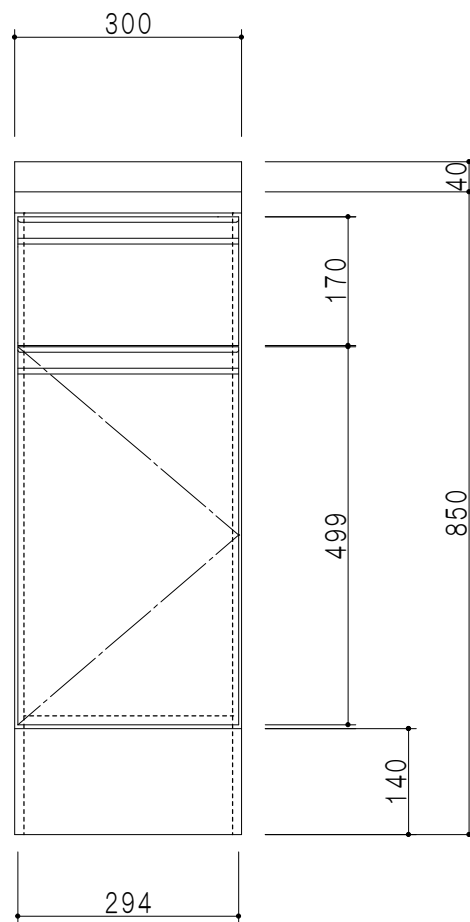
立面図
