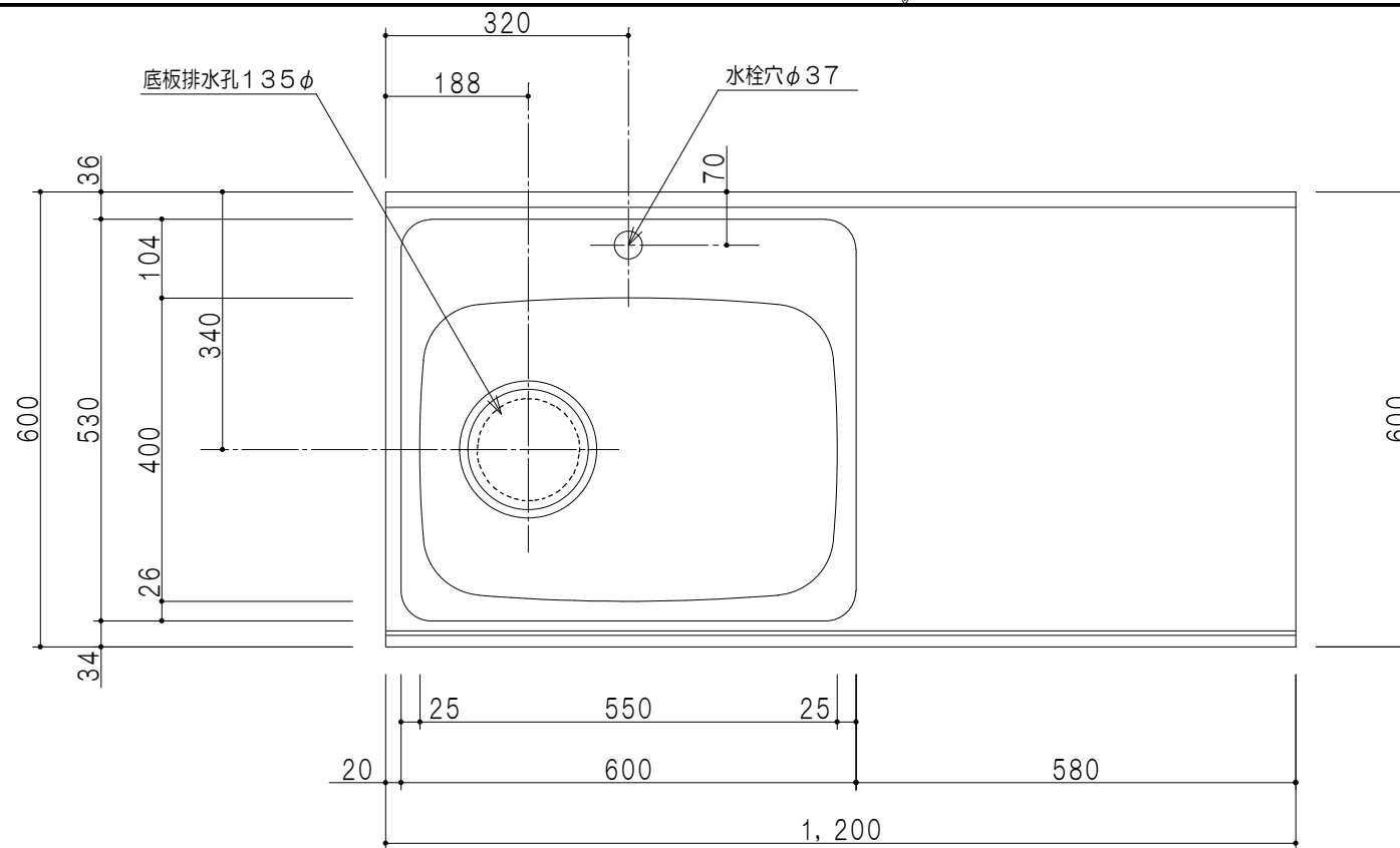
平面図
