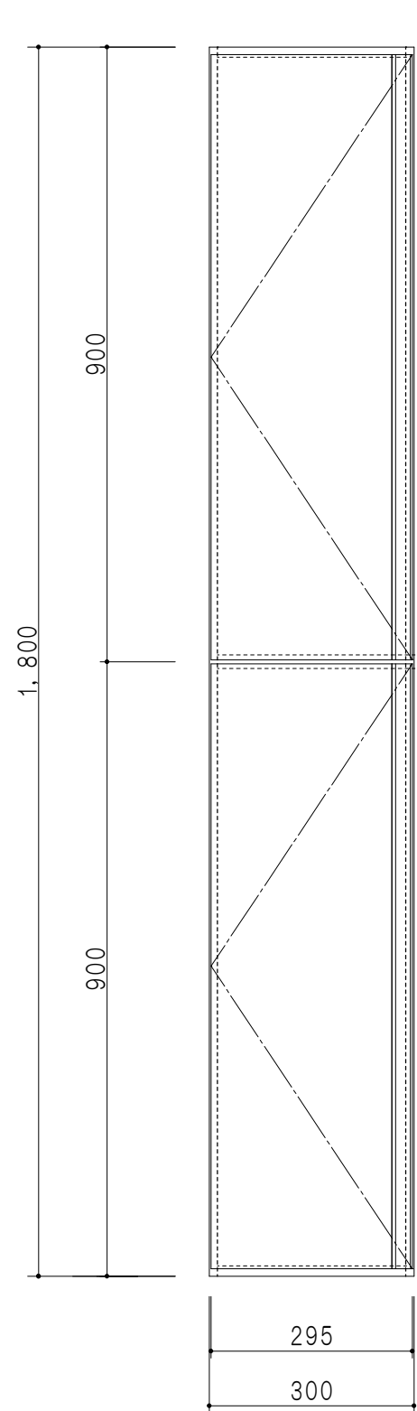
立面図
