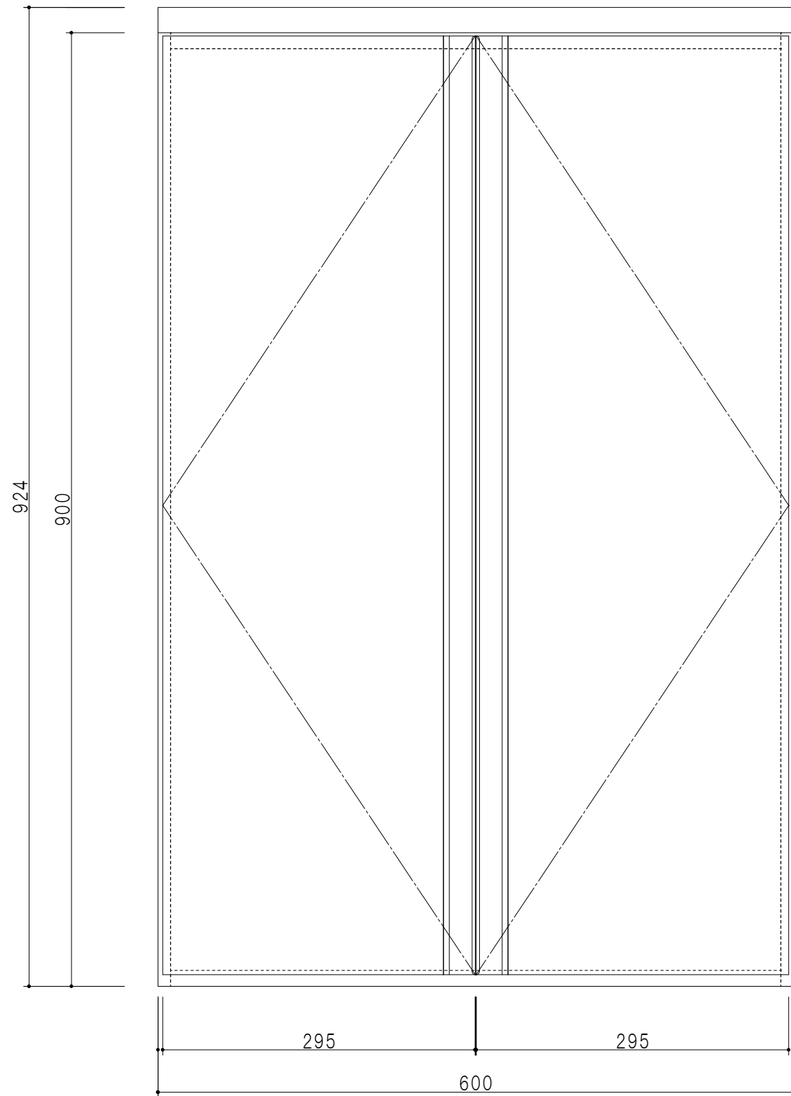
立面図
