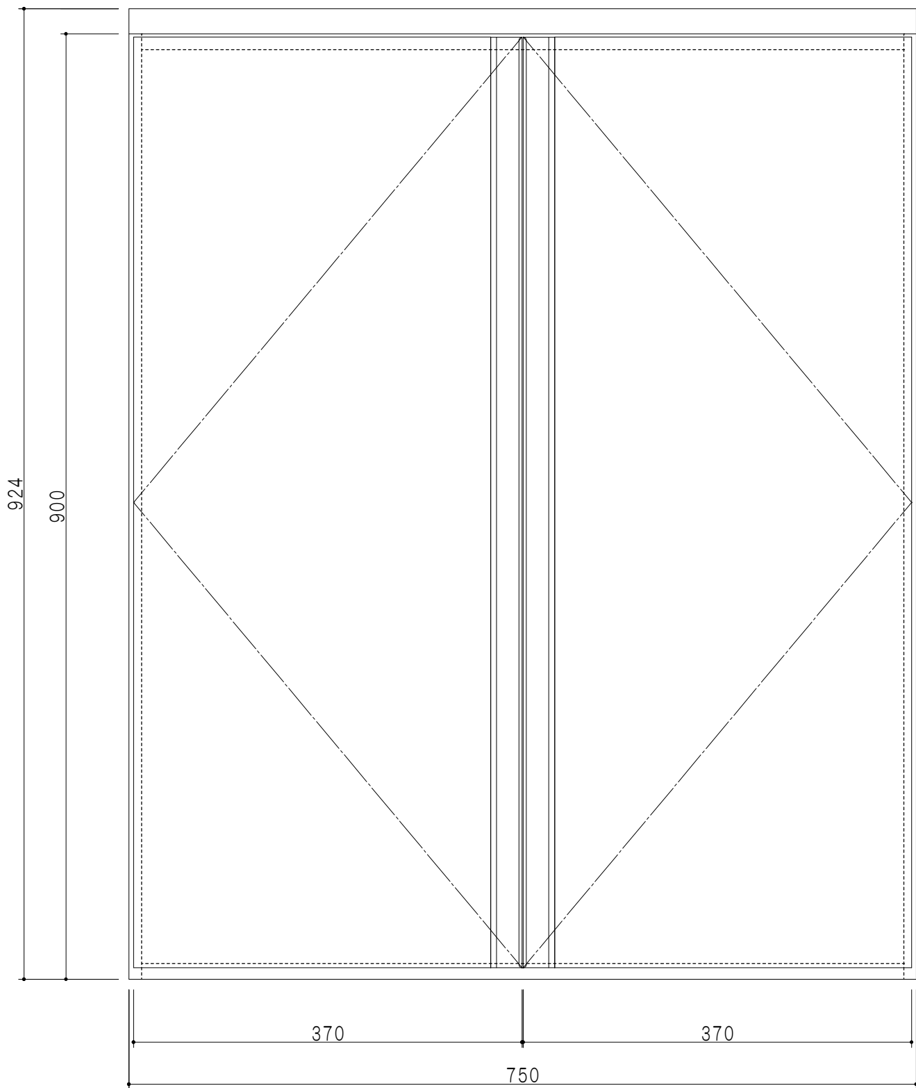
立面図
