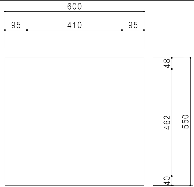
平面図
