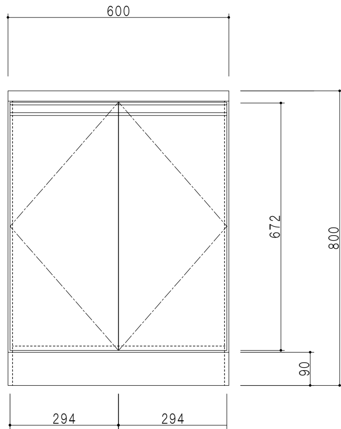
立面図
