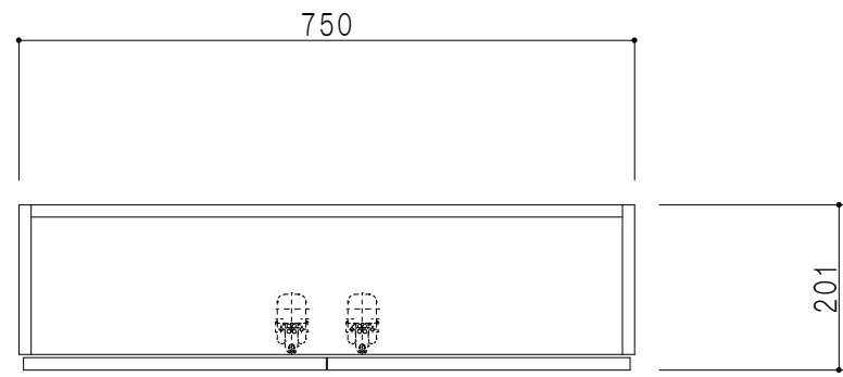
平面図
