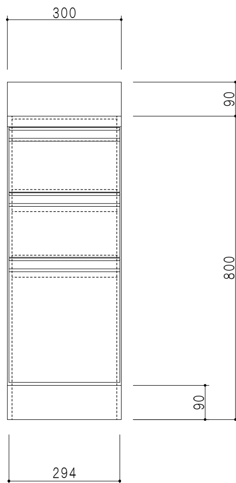
立面図
