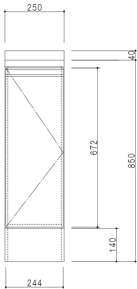
立面図
