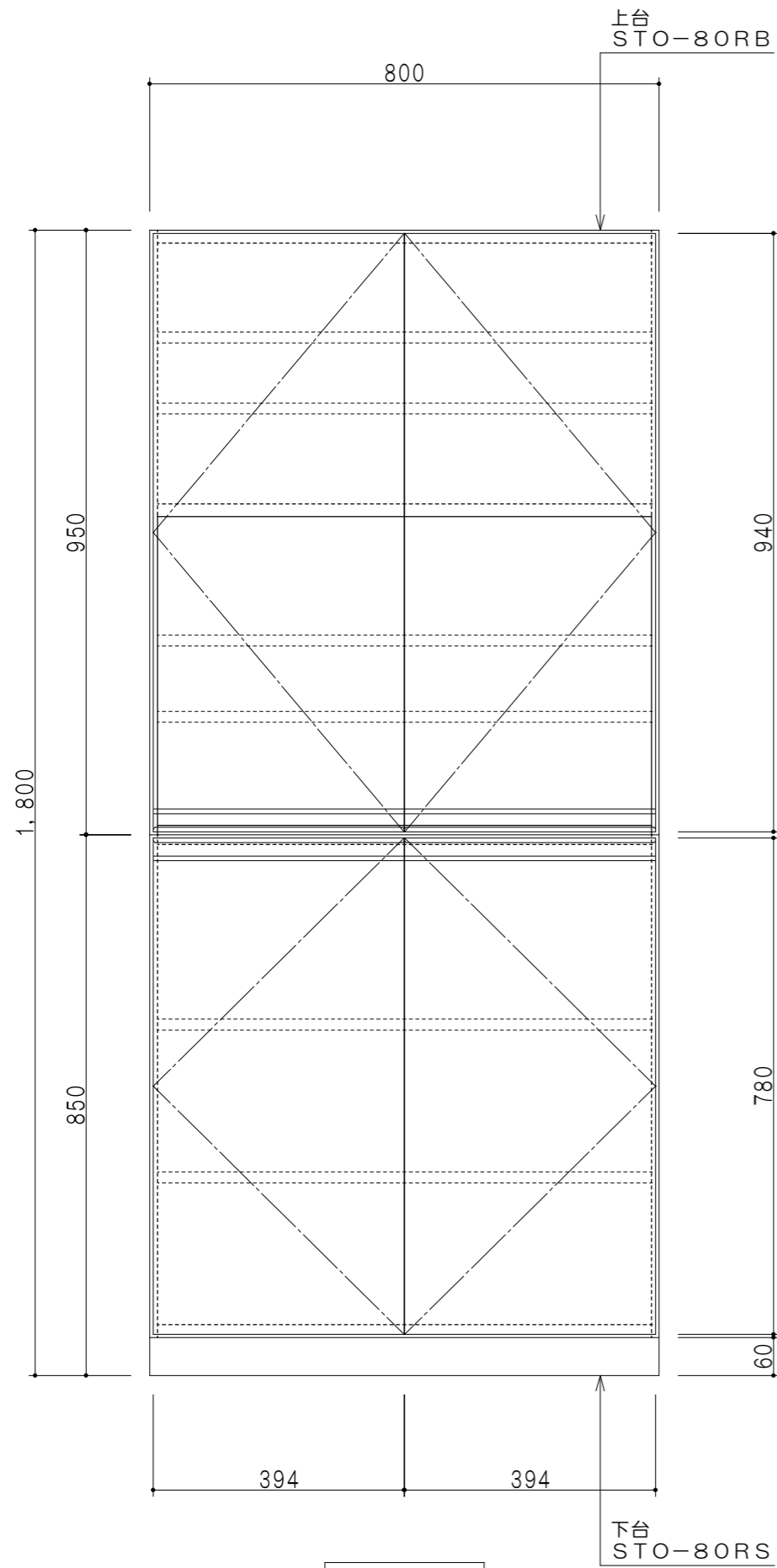
立面図
