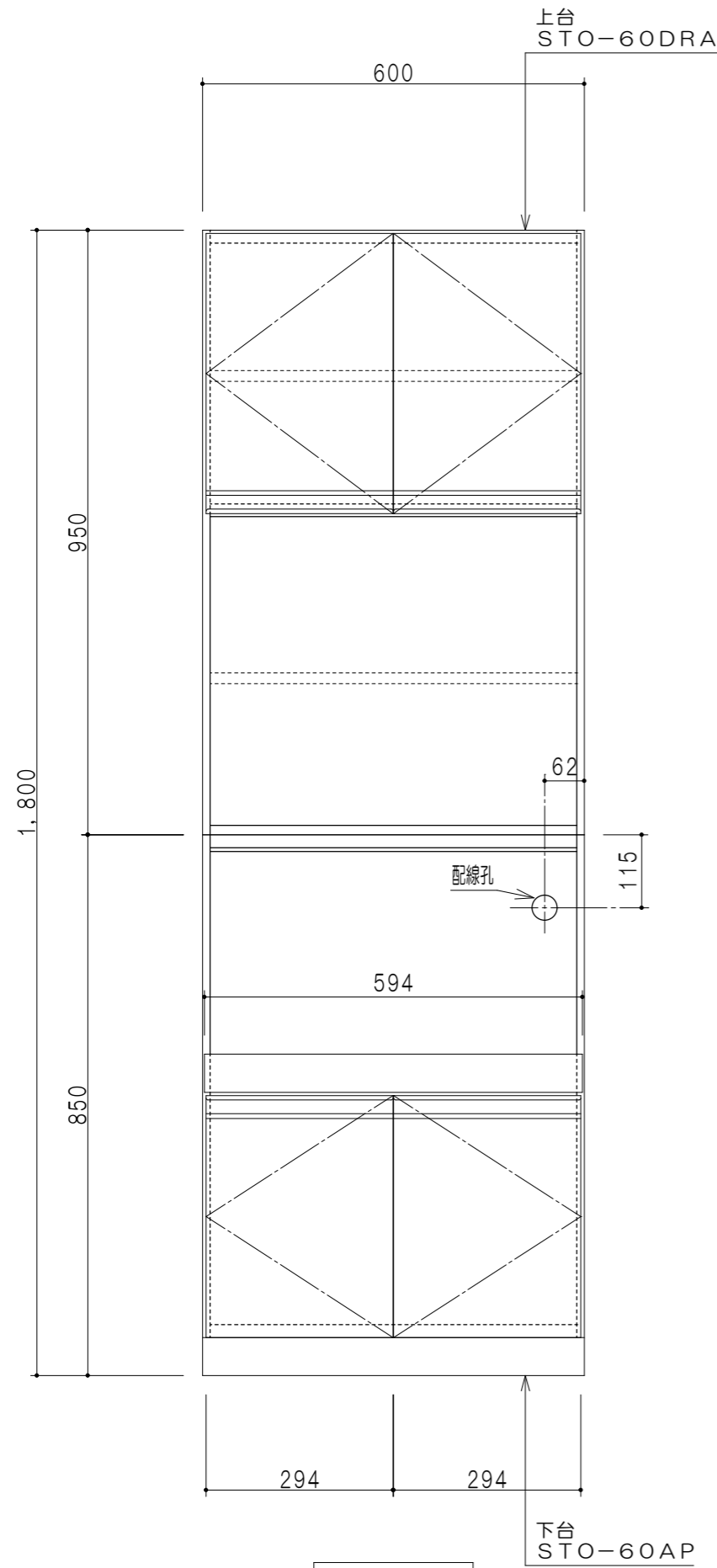
立面図
