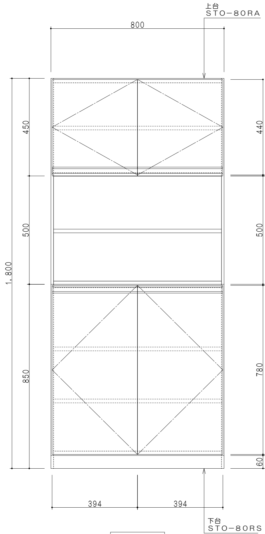
立面図
