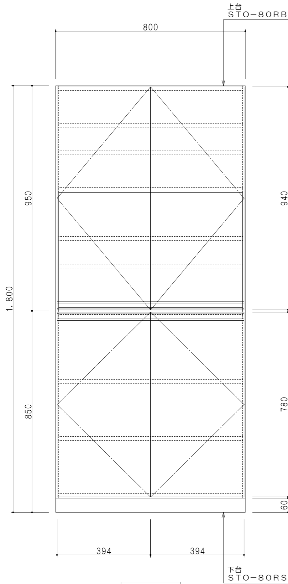
立面図
