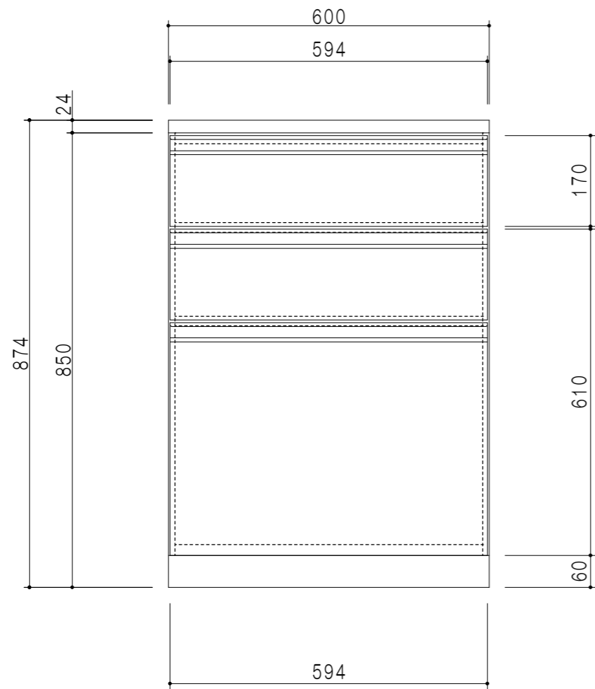
立面図
