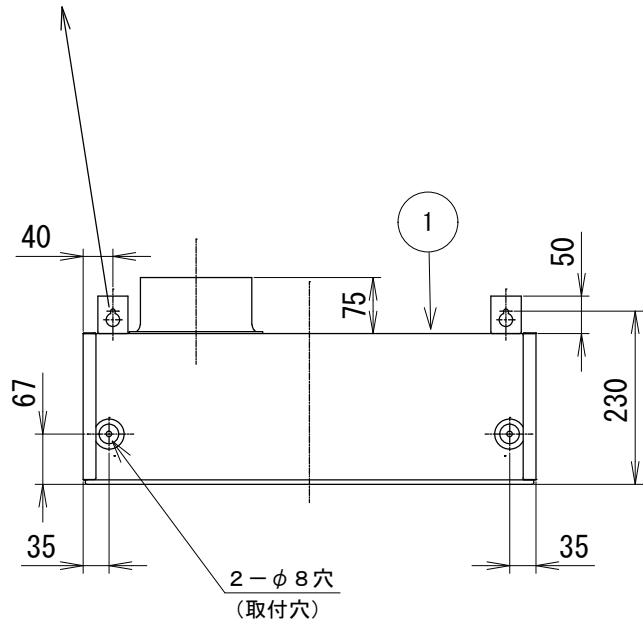
上部取付穴詳細
