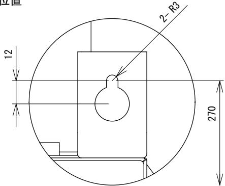
上部本体固定穴詳細図A
