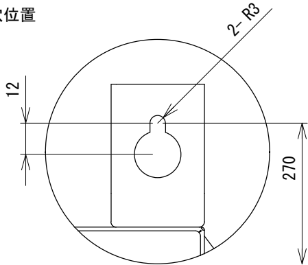
上部本体固定穴詳細図A
