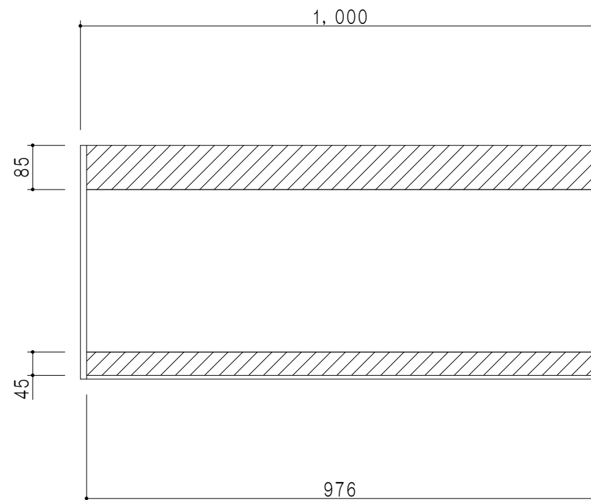
背面図
