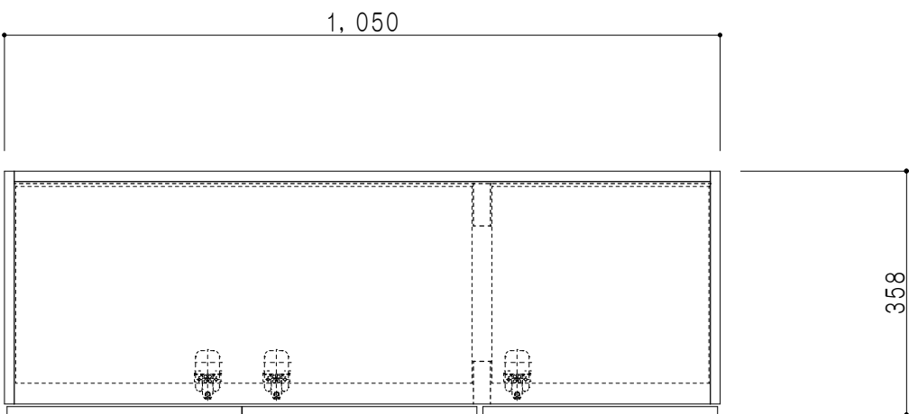
平面図
