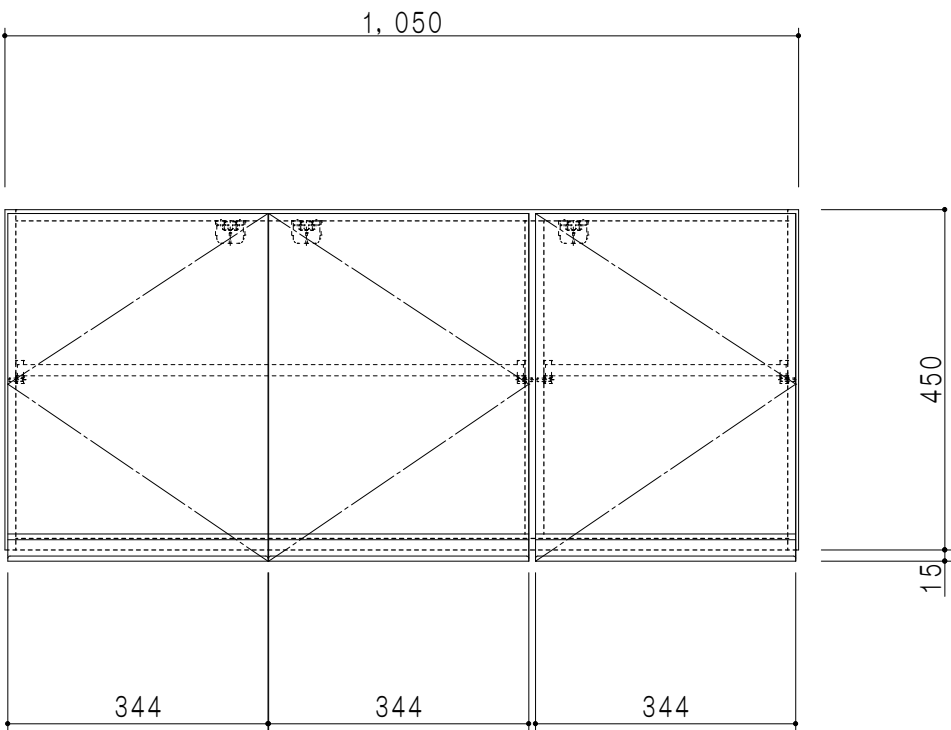
立面図
