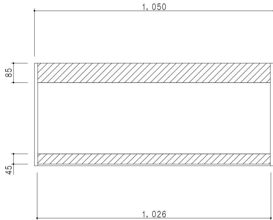
背面図
