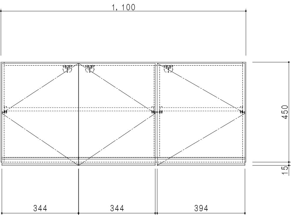
立面図
