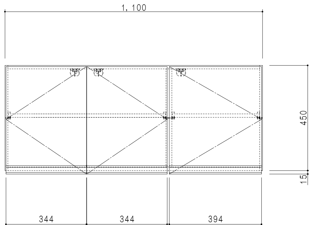
立面図
