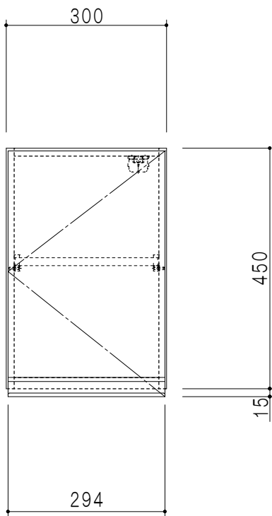
立面図
