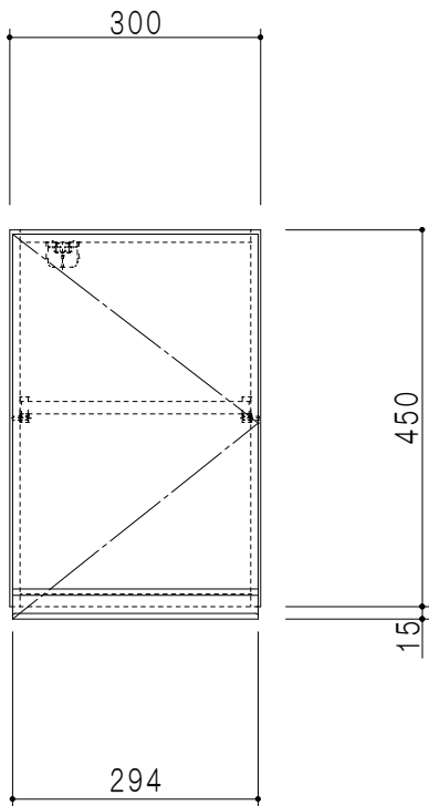
立面図
