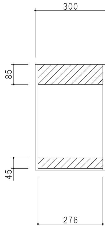
背面図
