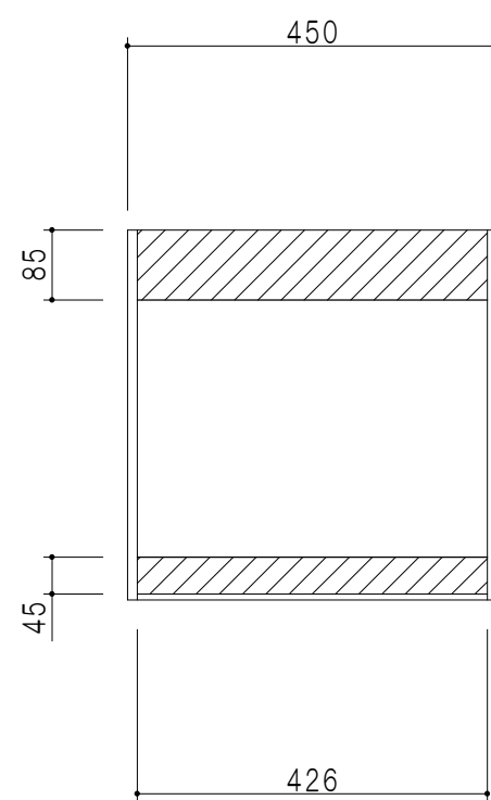
背面図
