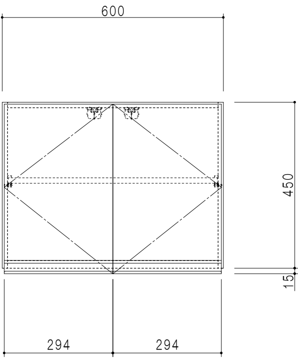
立面図
