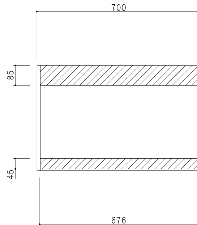
背面図
