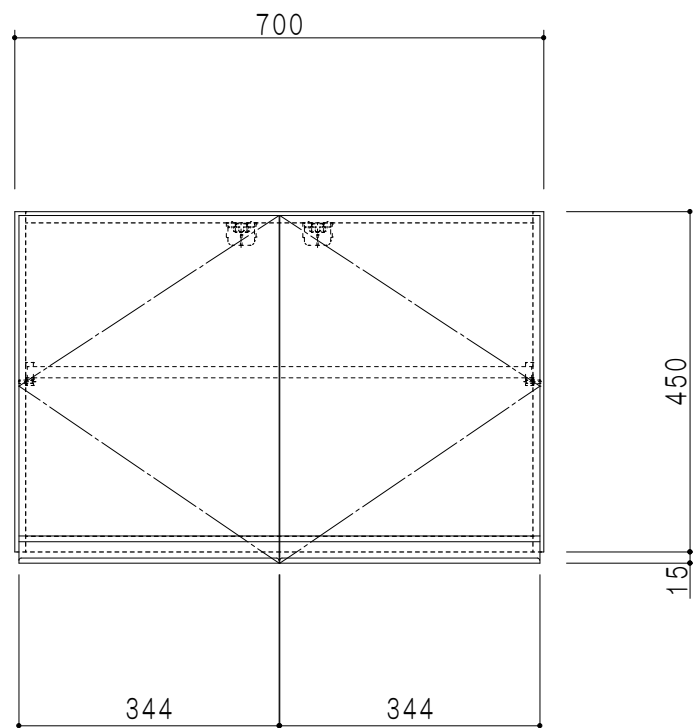
立面図
