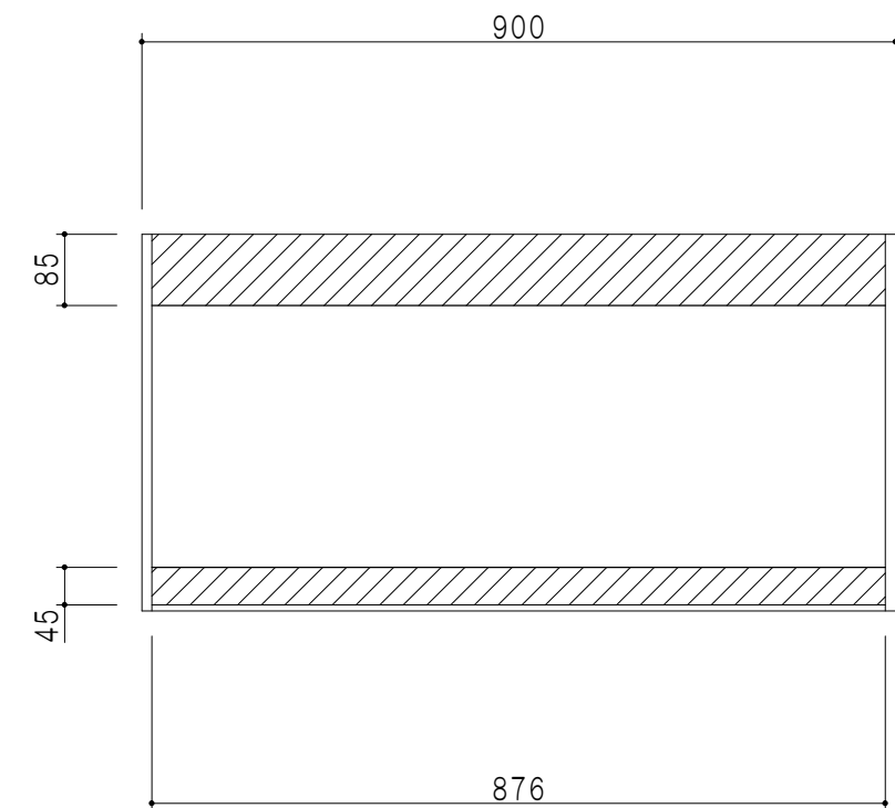
背面図
