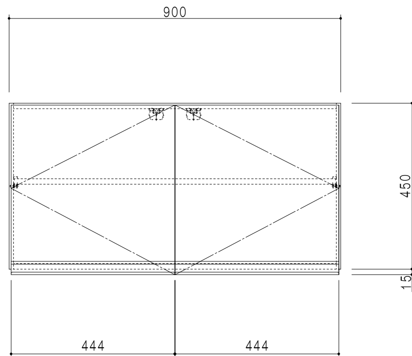
立面図
