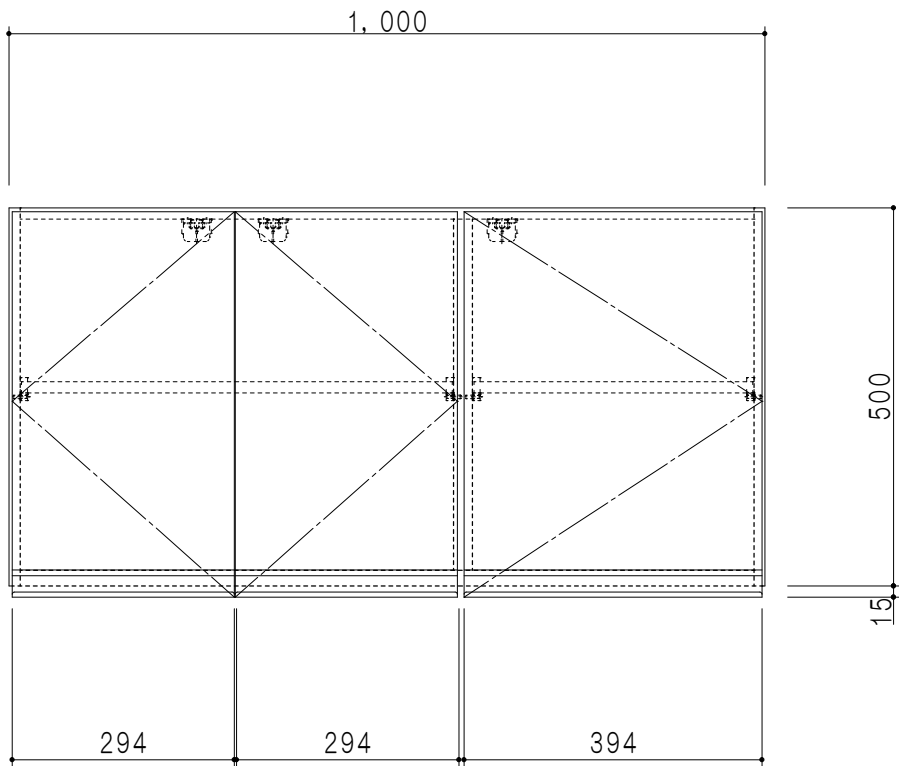
立面図
