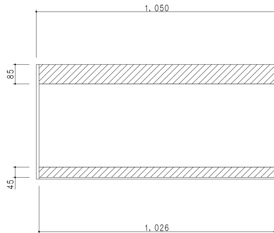
背面図
