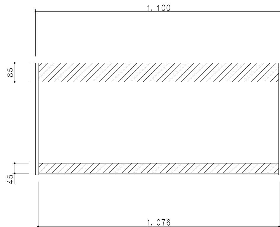
背面図
