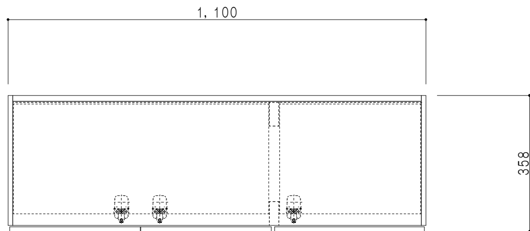
平面図
