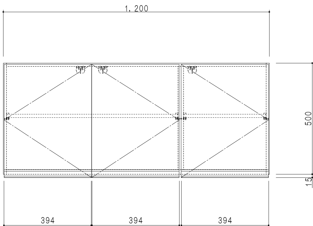
立面図
