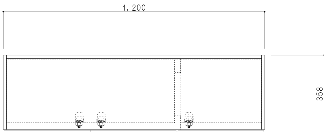
平面図
