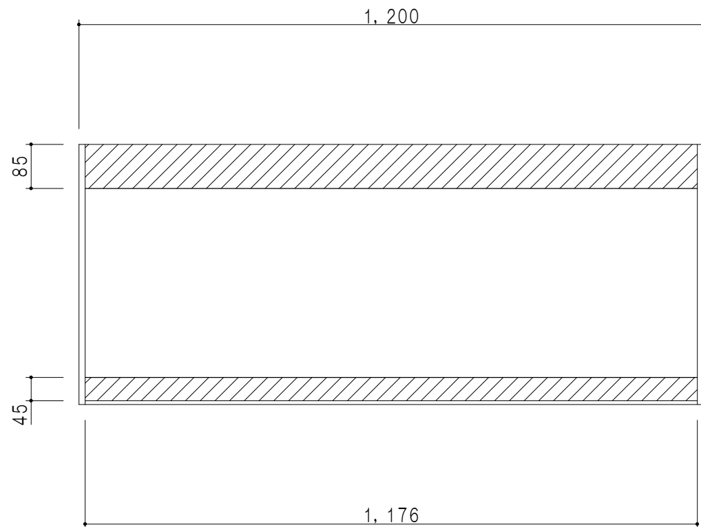
背面図
