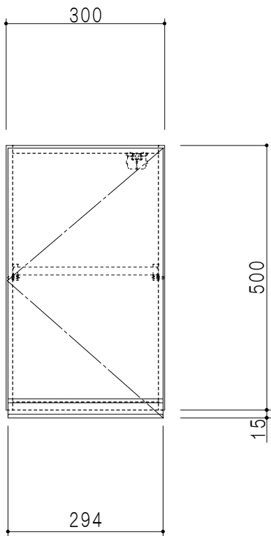
立面図
