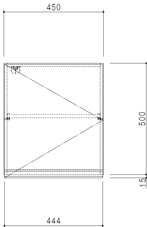
立面図
