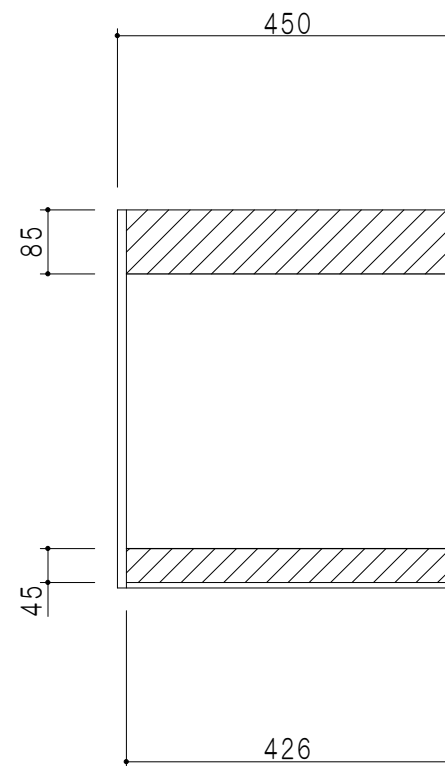
背面図
