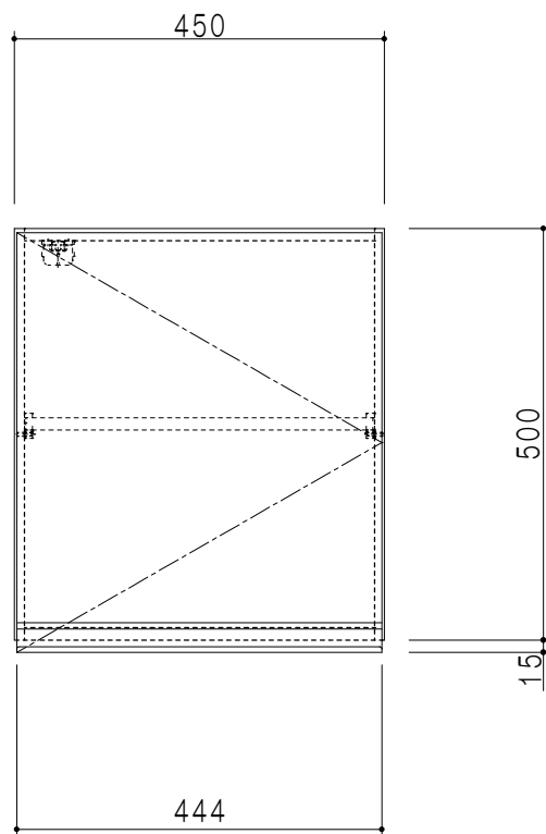
立面図
