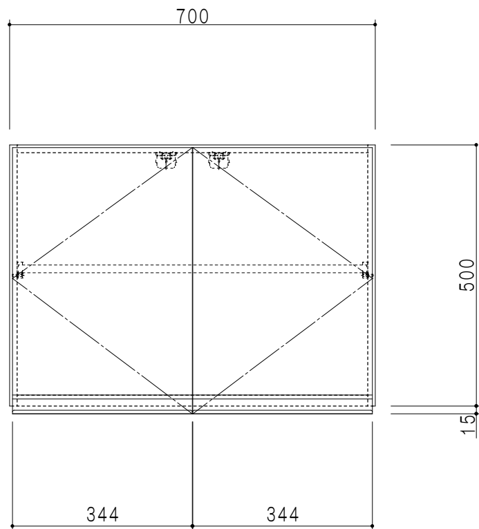
立面図
