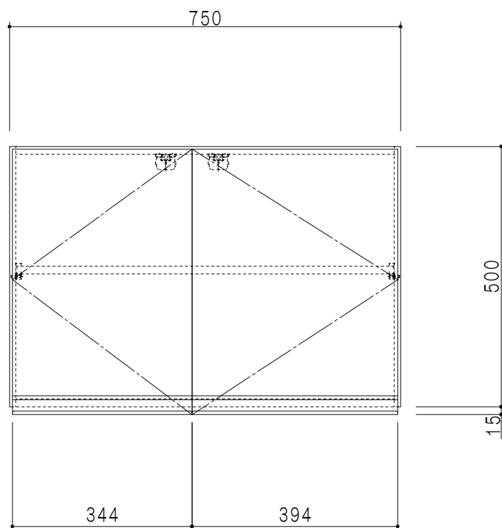
立面図
