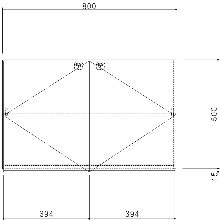
立面図
