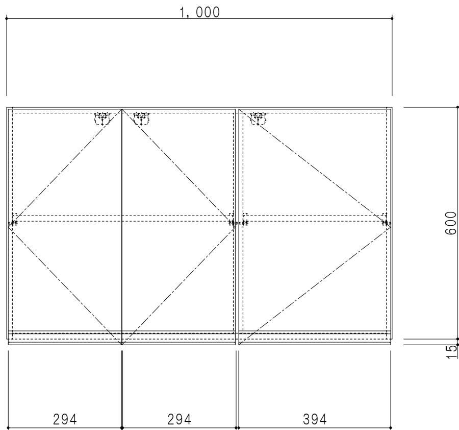
立面図
