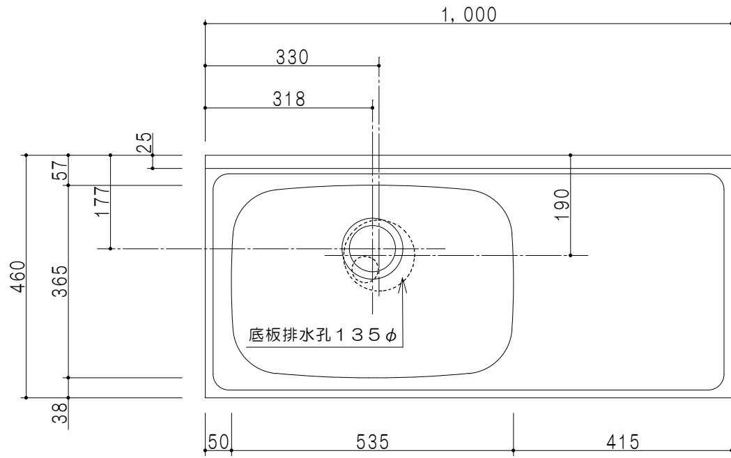
平面图
