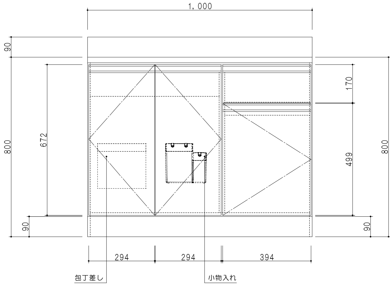
立面图
