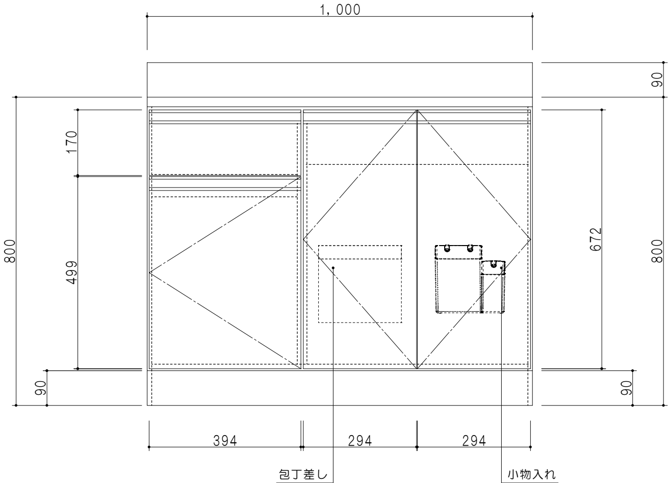
立面図
