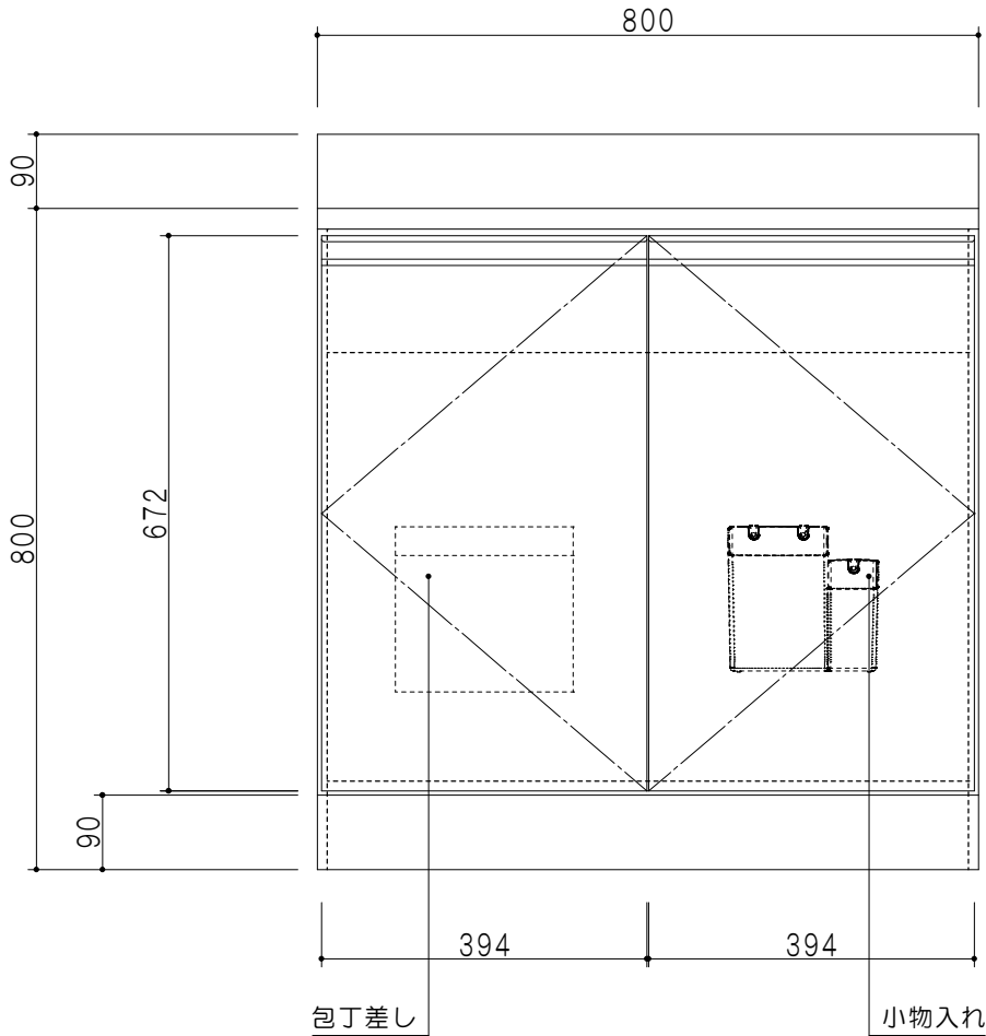
立面図
