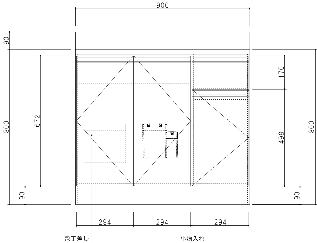
立面図
