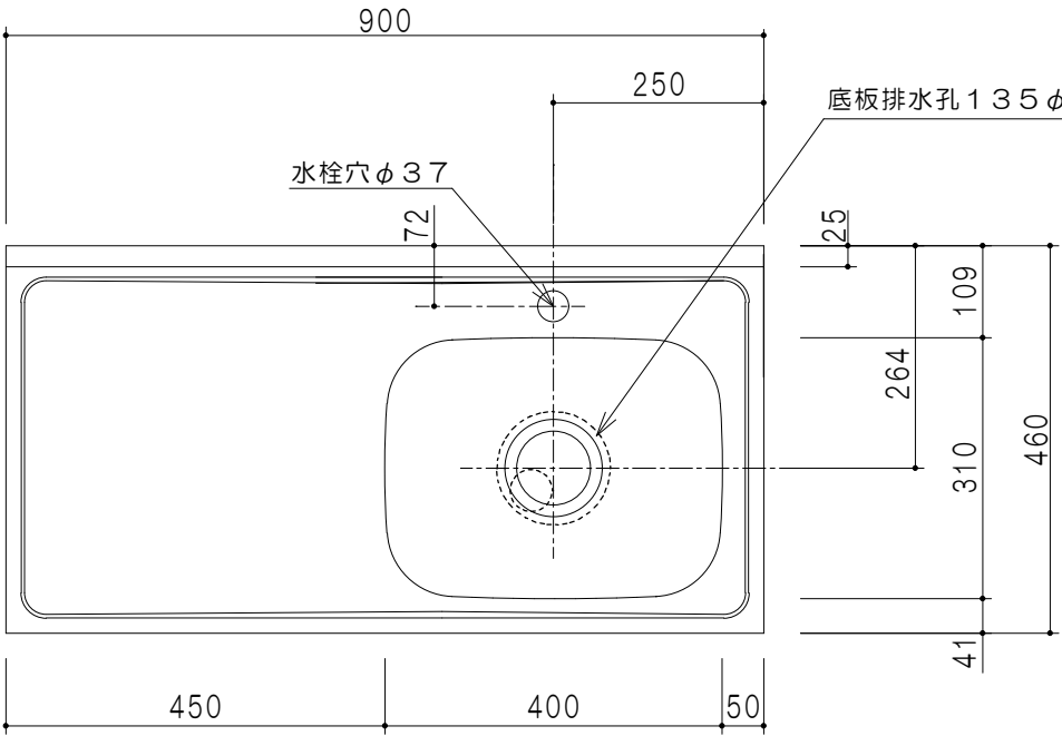
平面図
