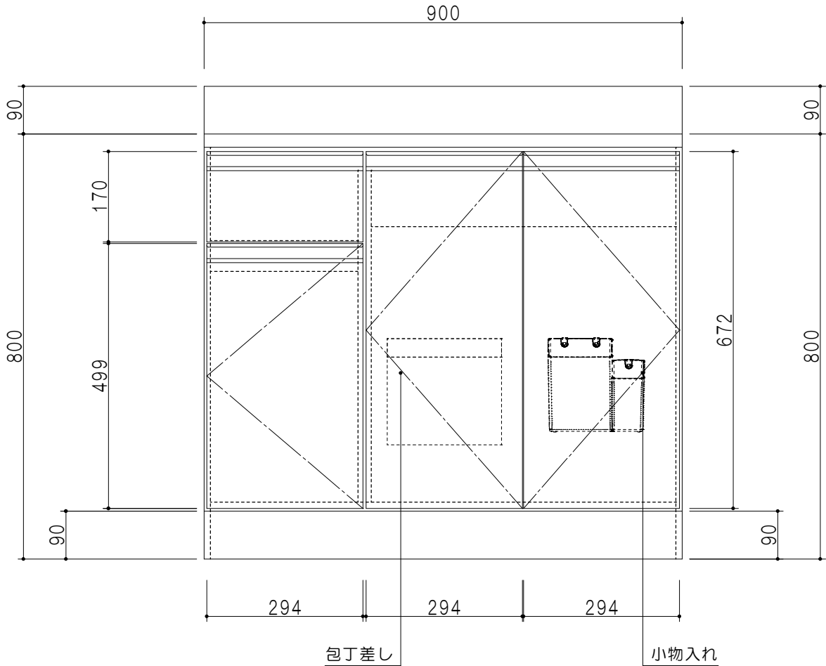
立面図
