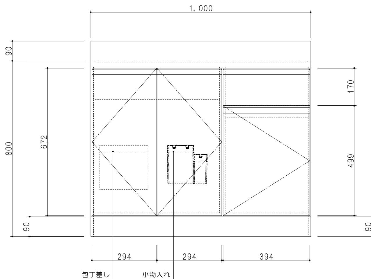
立面図
