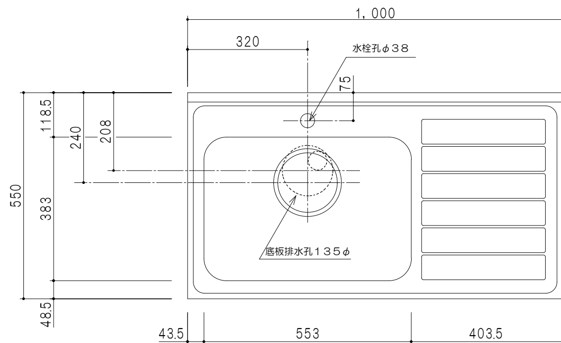
平面図
