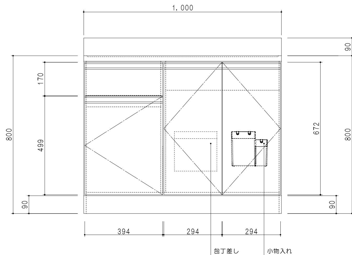
立面图
